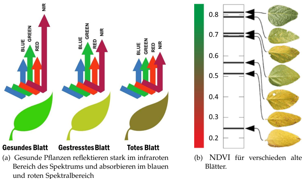
Abb. 5.8: Je gesünder eine Pflanze ist, desto höher ist die Reflexion im nahen Infrarotbereich. Bildquelle: http://physicsopenlab.org/2017/01/30/ndvi-index/
